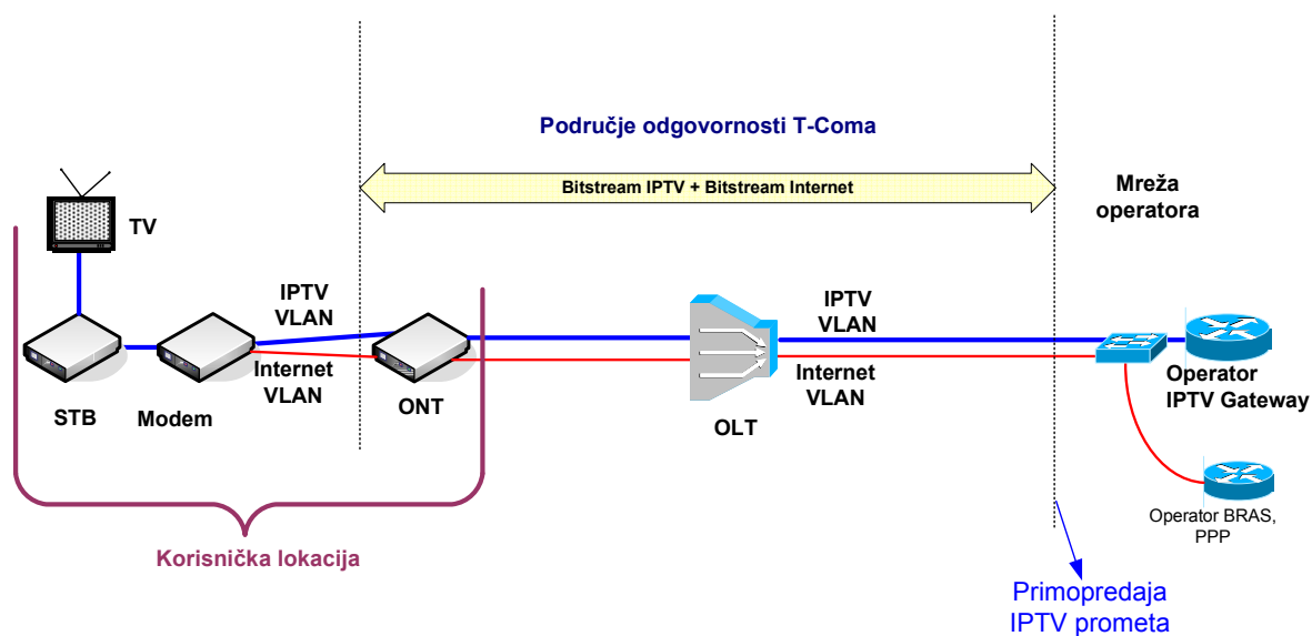
Slika 21. Veleprodajni širokopojsni pristup za pružanje IPTV usluge preko FTTH pristupa (GPON) na OLT razini
