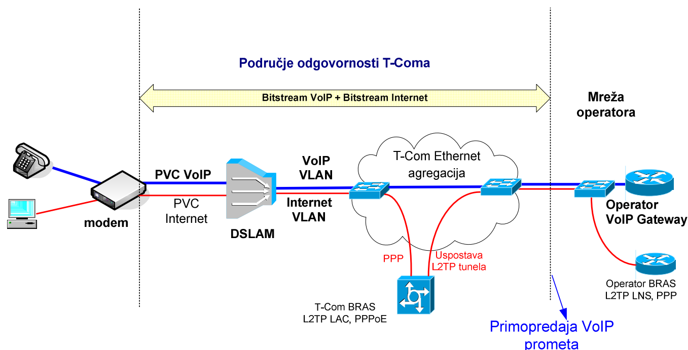
Slika 8. Realizacija posebnog virtualnog kanala za VoIP uslugu preko ADSL/VDSL pristupa (kod VDSL pristupa između modema i DSLAM-a koristi se odgovarajući VLAN)
