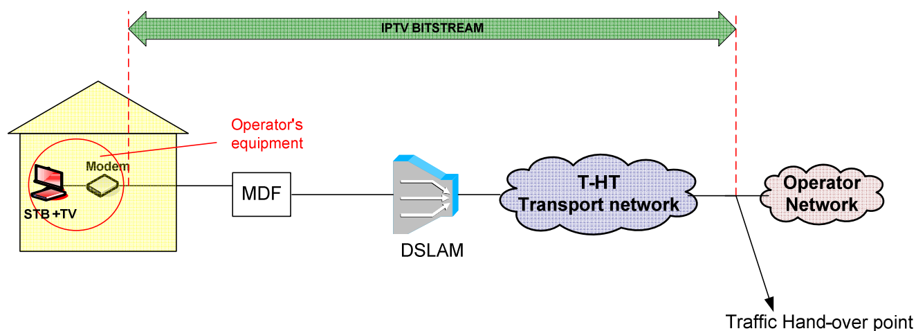
Slika 16. Koncept posebnog virtualnog kanala za IPTV uslugu u slučaju kada Krajnji korisnik ostvaruje Osnovni pristup mreži putem usluge Operatora korisnika
