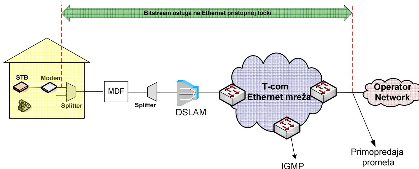
Slika 19. IPTV usluga na Ethernet razini putem ADSL/VDSL tehnologije u slučaju kada Krajnji korisnik ostvaruje Osnovni pristup mreži putem usluge T-Coma
