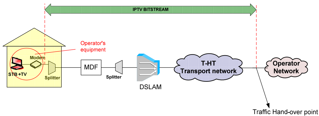
Slika 15. Koncept posebnog virtualnog kanala za IPTV uslugu u slučaju kada Krajnji korisnik ostvaruje Osnovni pristup mreži putem usluge T-Coma
