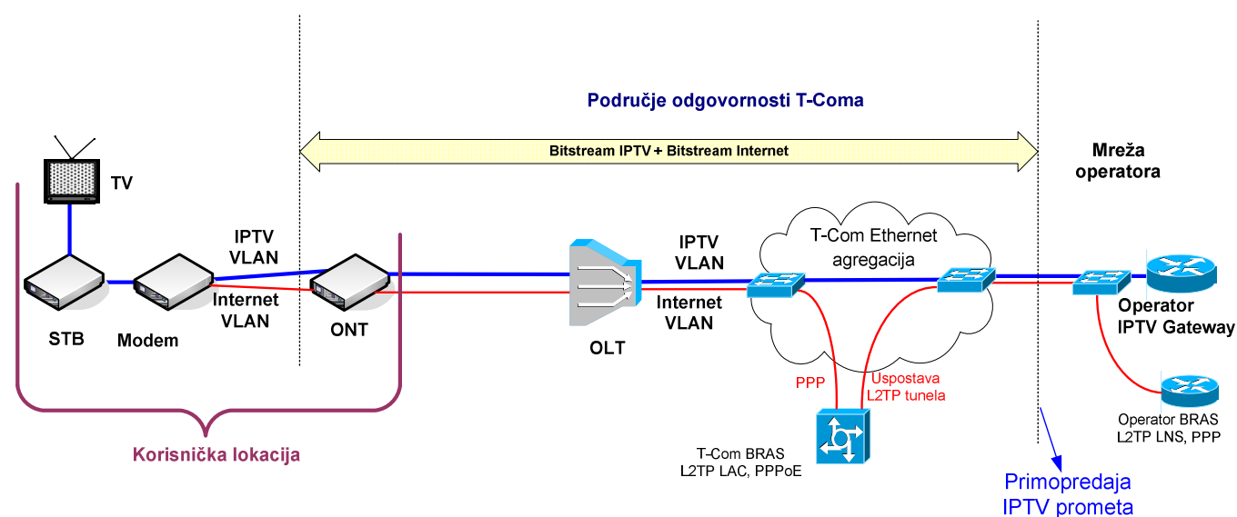
Slika 18. Realizacija posebnog virtualnog kanala za IPTV uslugu preko FTTH pristupa (GPON)
