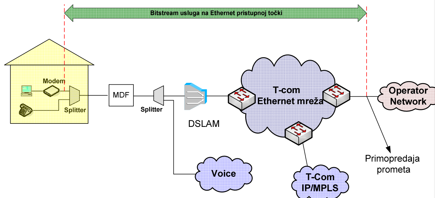
Slika 10. Veleprodajni širokopojsni pristup za pružanje VoIP usluge na Ethernet razini u slučaju kada Krajnji korisnik ostvaruje Osnovni pristup mreži putem usluge T-Coma
