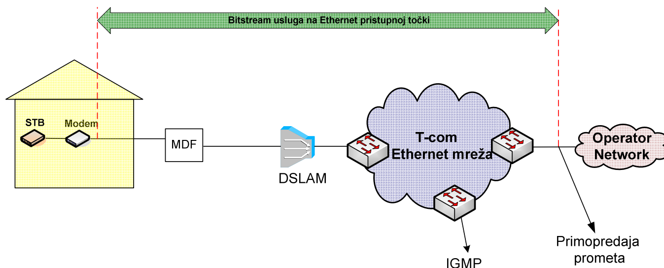
Slika 20. IPTV usluga na Ethernet razini putem ADSL/VDSL tehnologije u slučaju kada Krajnji korisnik ostvaruje Osnovni pristup mreži putem usluge Operatora korisnika
