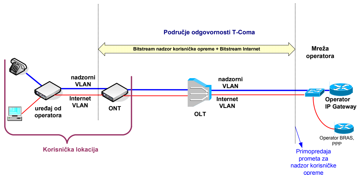
Slika 22. Veleprodajni širokopojasni pristup za pružanje usluge nadzora korisničke opreme preko FTTH pristupa (GPON) na OLT razini
