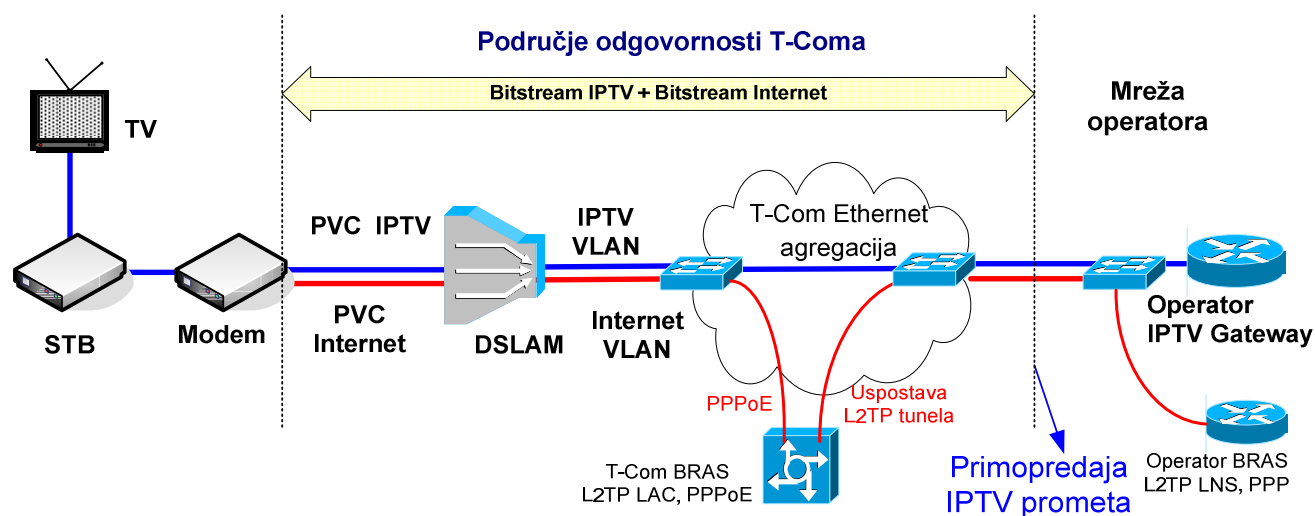
Slika 17. Realizacija posebnog virtualnog kanala za IPTV uslugu preko ADSL/VDSL pristupa (kod VDSL pristupa između modema i DSLAM-a koristi se odgovarajući VLAN)
